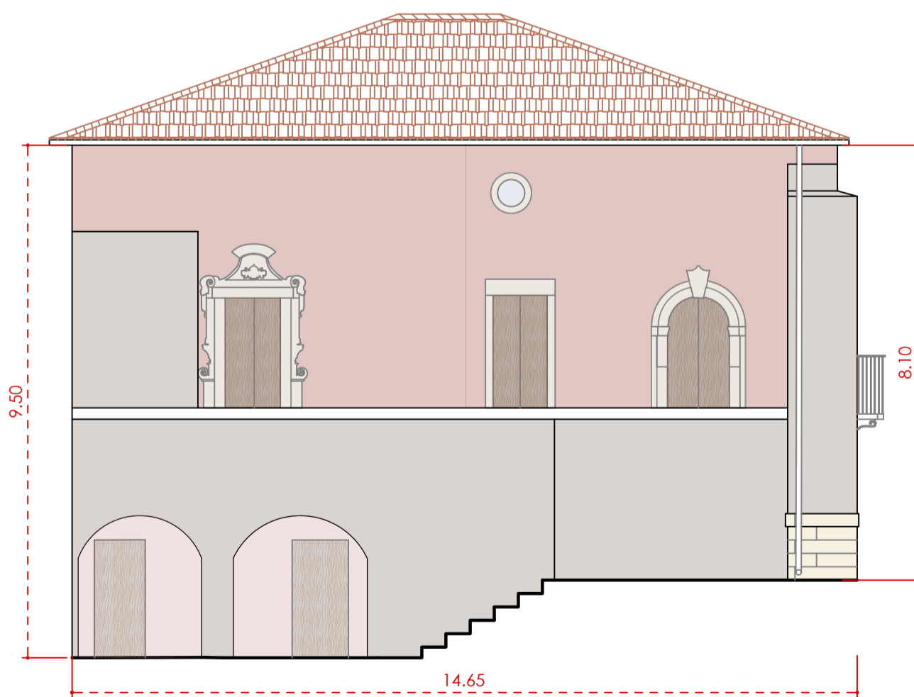
PROGETTO PROSPETTO LATO INGRESSO (Rapp. 1:100)
