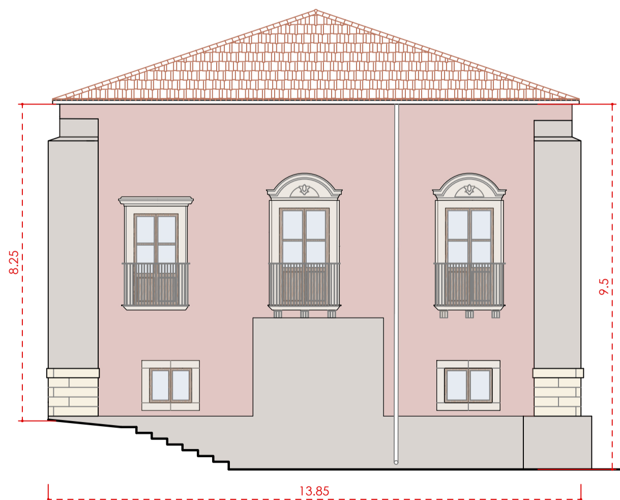
PROGETTO PROSPETTO LATO CHIESA (Rapp. 1:100)
